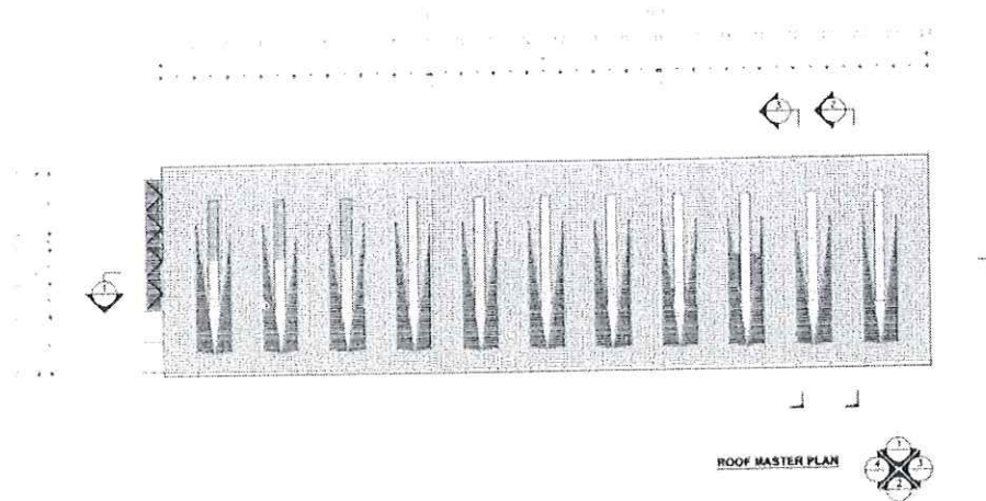
รูปภาพที่ 1 Layout plan ศูนย์ซ่อมบำรุงรถไฟฟ้า CT Depot Main workshop
